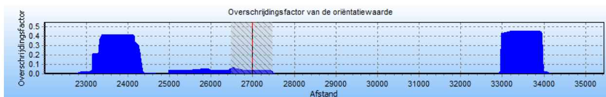
Figuur 68 Overschrijding van het groepsrisico als functie van de stationing van de A-515, gedeelte van de leiding nabij Westvaartpark. De verticale rode lijn toont het middelpunt van de kilometer waarover de FN-curve in de volgende twee figuren is berekend. De stationing neemt toe in oost-westrichting.
