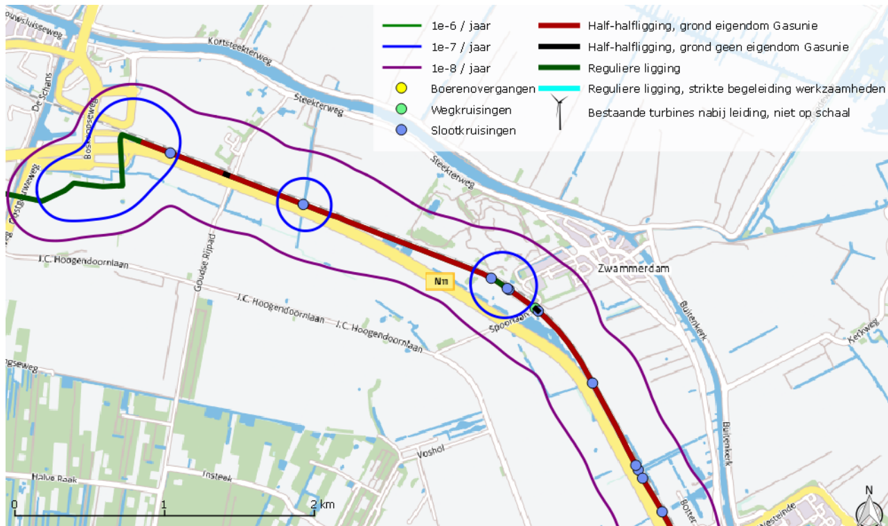
Figuur 38: Plaatsgebonden risico van de gastransportleiding A-515, derde gedeelte, berekend met PIPESAFE. Het PR is overal in dit gebied kleiner dan 10^{-6} per jaar.
