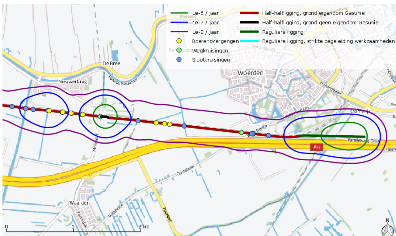
Figuur 18: Plaatsgebonden risico van de gastransportleiding A-515, meest oostelijk gedeelte, berekend met CAROLA. Het PR is overal in dit gebied kleiner dan 10^{-5} per jaar.
