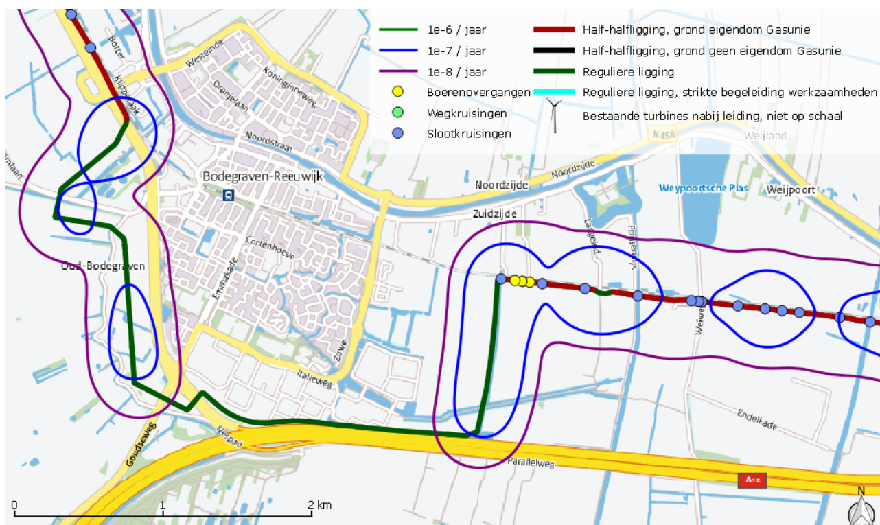
Figuur 37: Plaatsgebonden risico van de gastransportleiding A-515, tweede gedeelte, berekend met PIPESAFE. Het PR is overal in dit gebied kleiner dan 10^{-6} per jaar.
