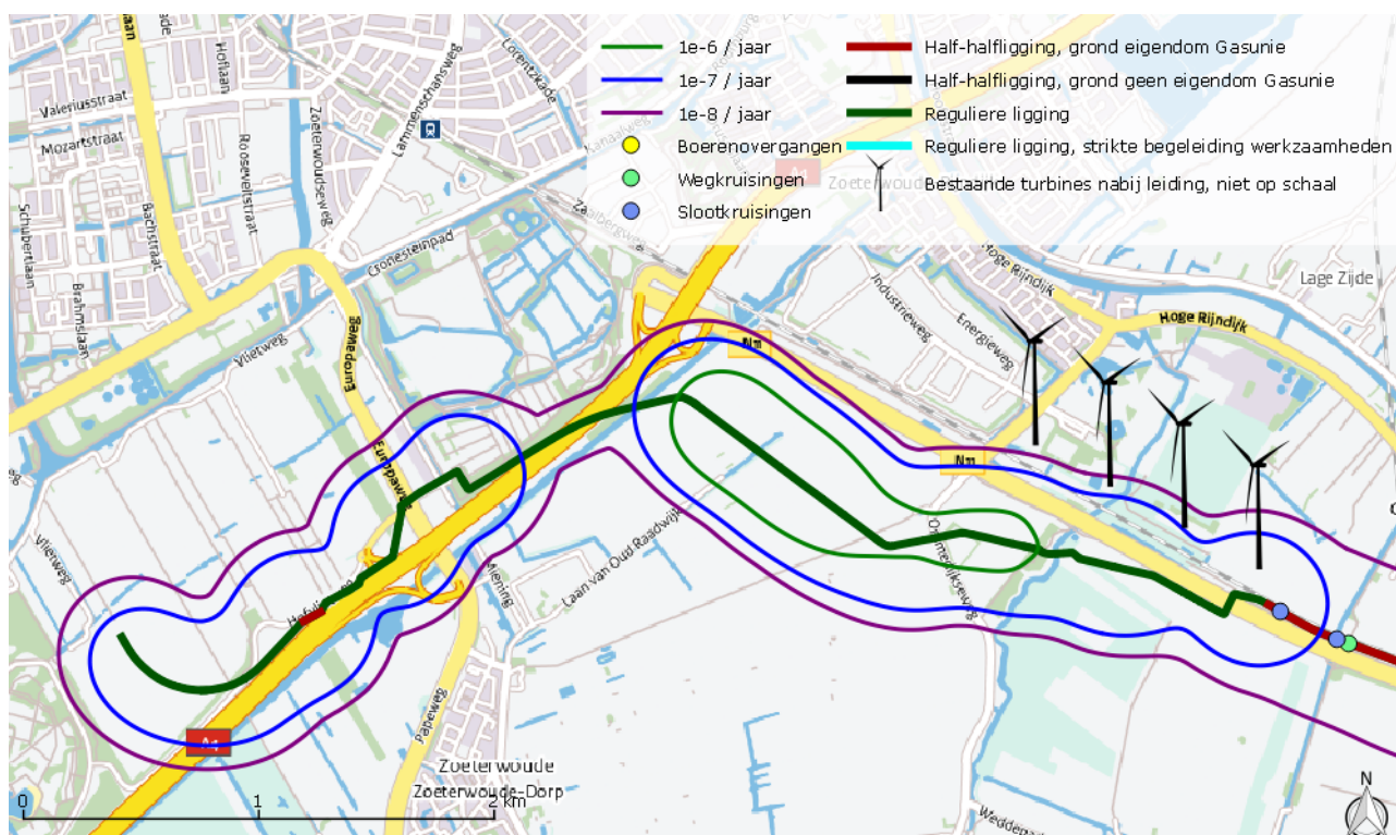
Figuur 41: Plaatsgebonden risico van de gastransportleiding A-515, meest westelijke gedeelte, berekend met PIPESAFE. Het PR is overal in dit gebied kleiner dan 10^{-5} per jaar.
