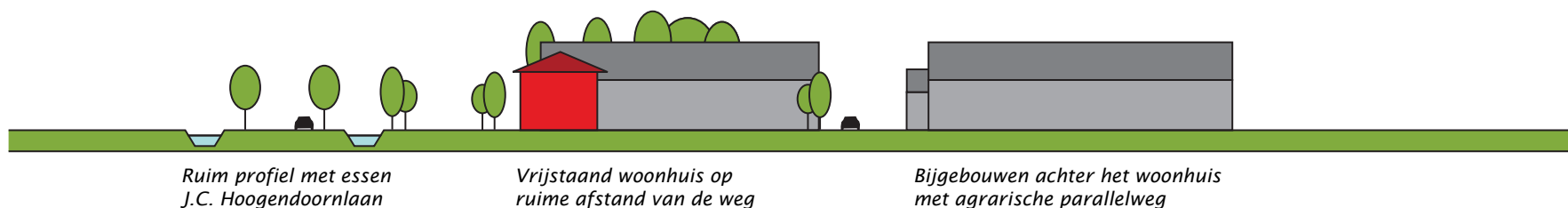
Principedoorsnede J.C. Hoogendoornlaan
