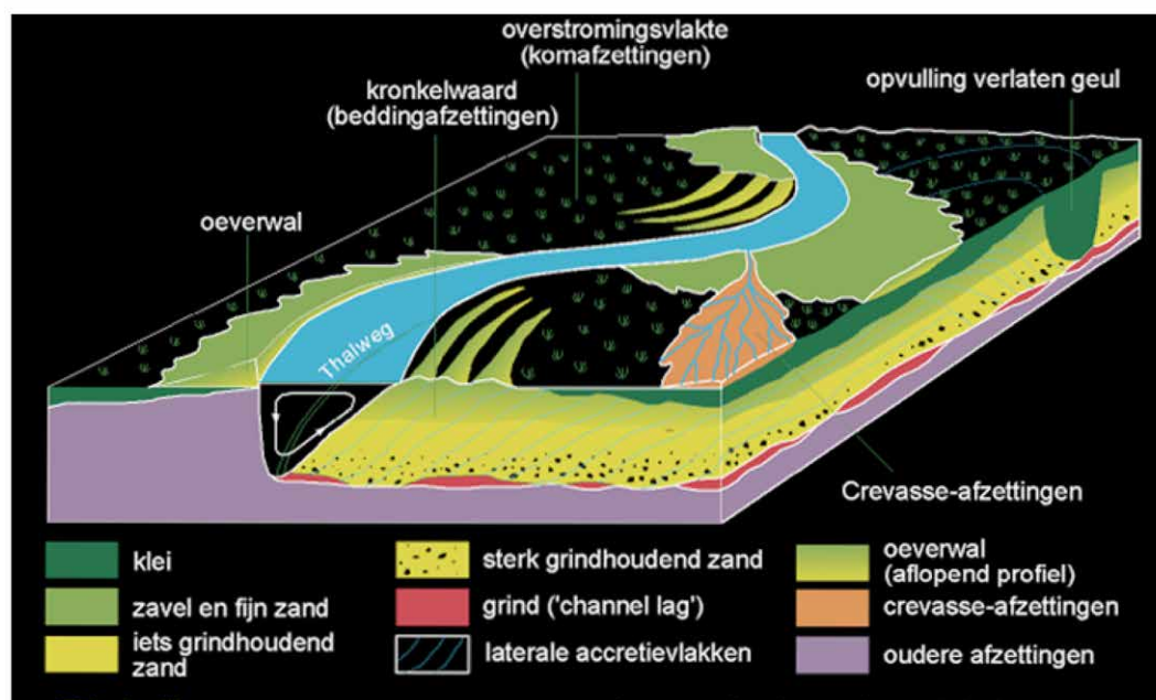
Afb. 2.1. Blokdigram van een meanderende laaglandrivier, Berendse 2011.
