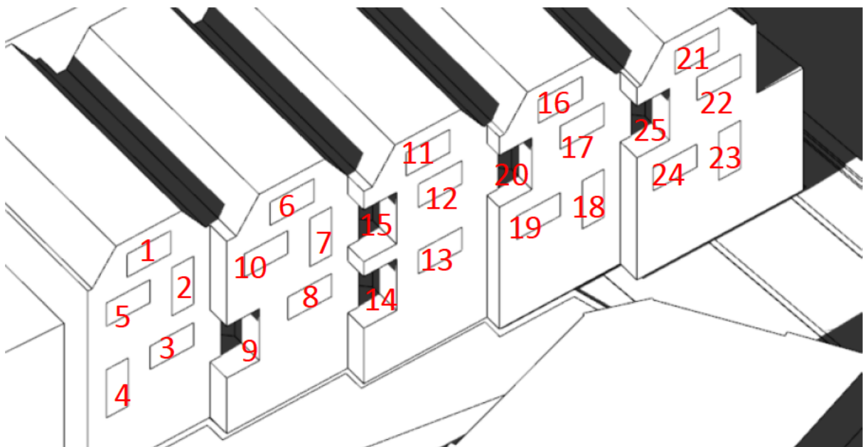
Figuur 25: Tweede gevel aanzicht Van Manderslootstraat inclusief raam nummering, 3D model.
