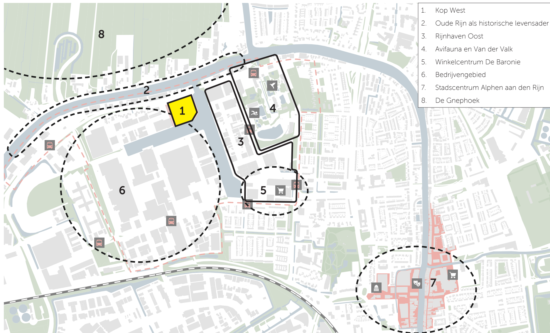
Stedenbouwkundig plan Havenfront / Rijnhaven Oost
